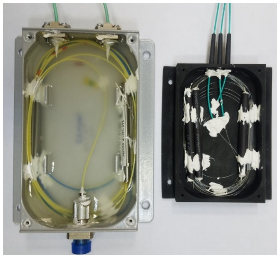
Рис. Монтаж двухкаскадного мультиплексора 1310/1550 на сварных ответвителях: а – с R_{\min} = 30 мм; б – с R_{\min} = 20 мм; использовалось ОВ, прошедшее 1 % proof test (см. табл. 4)
